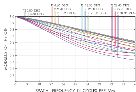
OPT-F3528-29M
