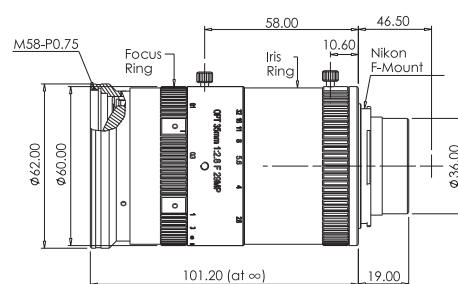
2.OPT-F3528-29M
