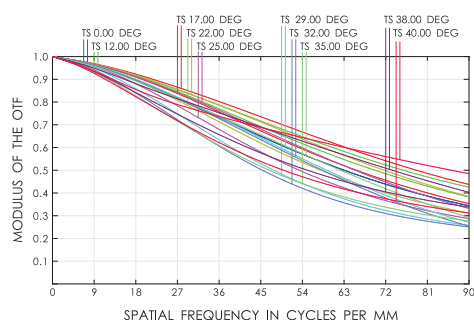
OPT-F2528-29M
