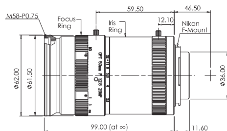
3.OPT-F5028-29M
