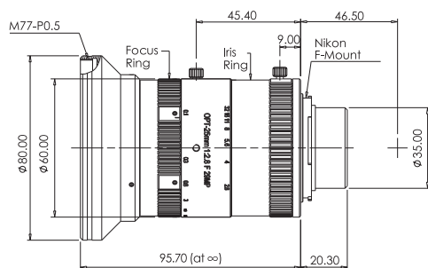
1.OPT-F2528-29M
