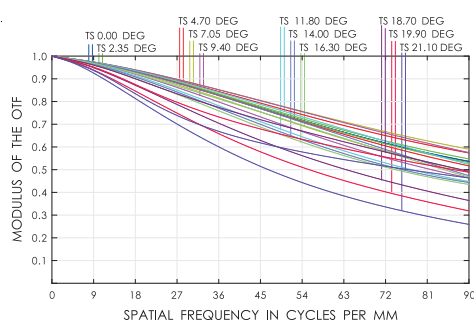
OPT-F5028-29M
